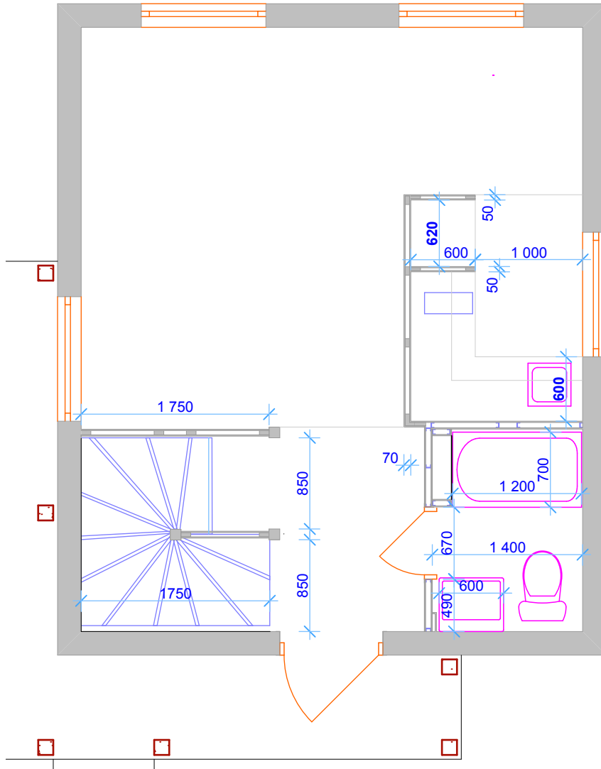
План 1 этажа
