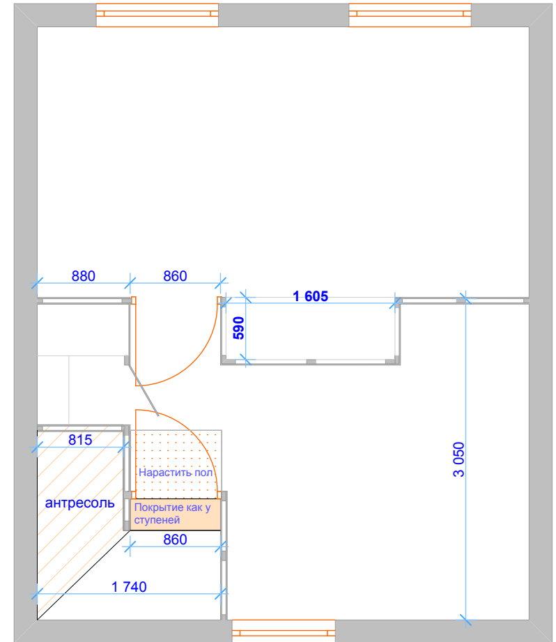
План мансарды
