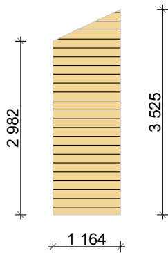
Фасад 1-4
