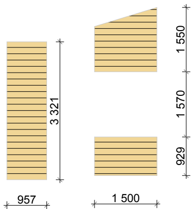
Фасад Е-А
