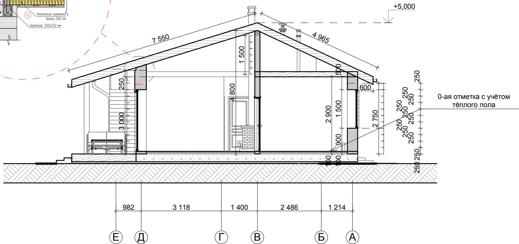
Разрез 2-2
