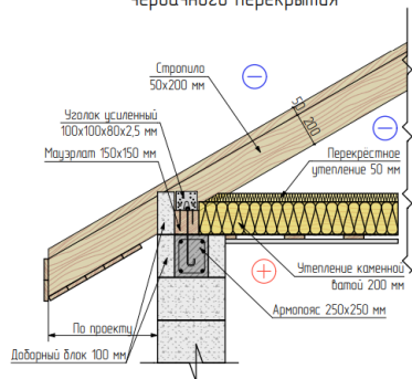
Узел 1 Опираие деревянных балок чердачного перекрытия
