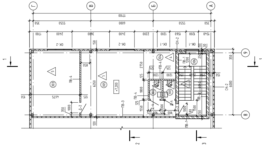
План на отм. +7,200
