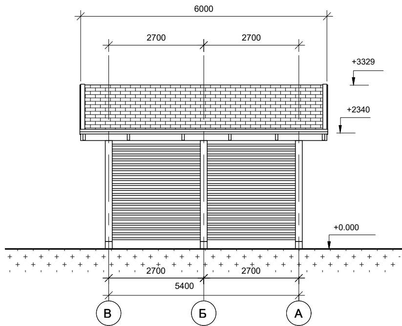
Фасад В-А
