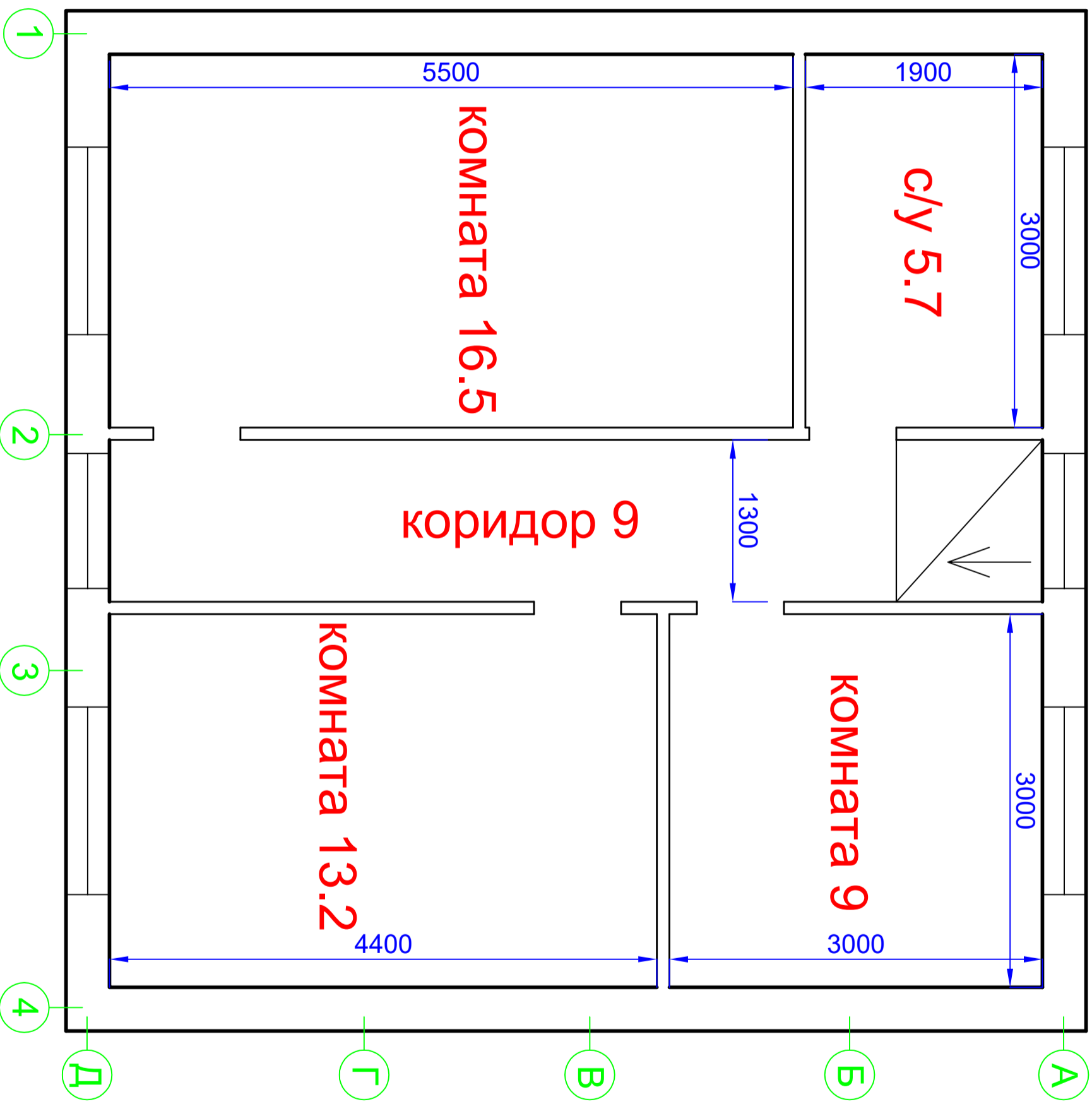
ПЛАНІРОВКА 2 ЕТАЖА
