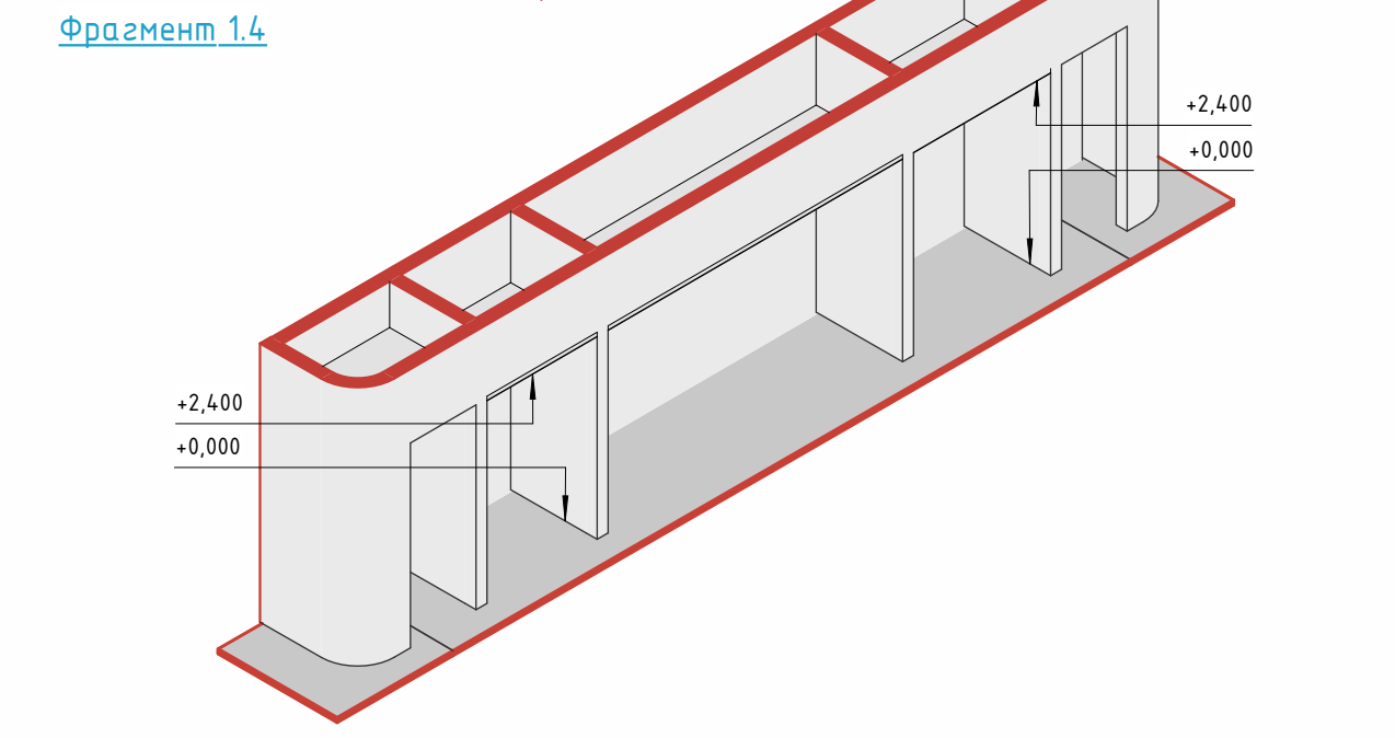
М.1.3 - М.1.3
