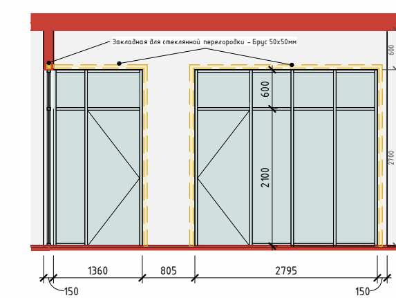
М.1.3 - М.1.3
