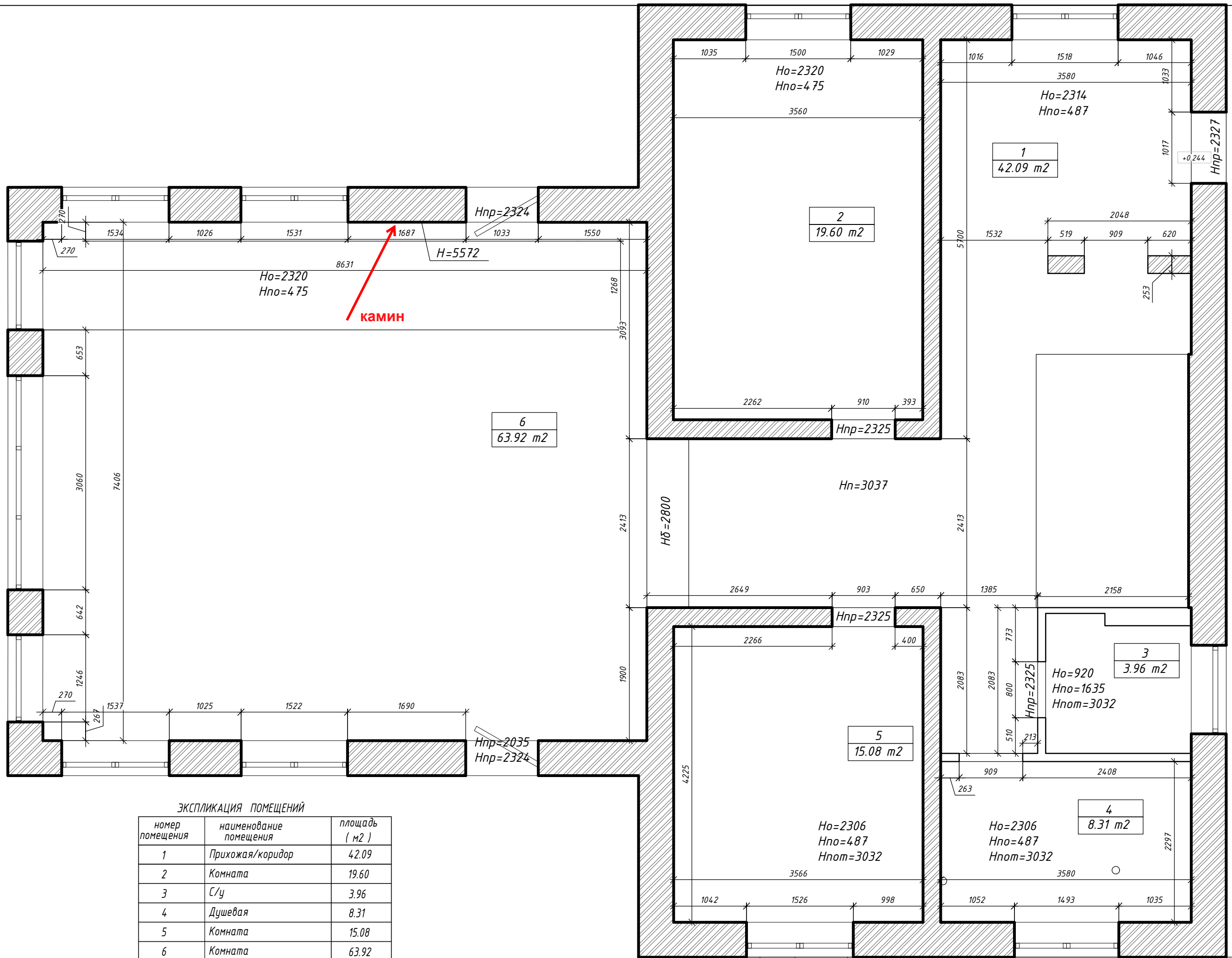
Обмерный план 1 этажа
